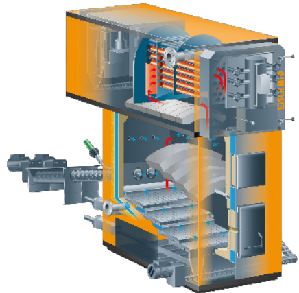
FIGURA 2 - Sinistra: generatore termico a combustione inversa per legna in tronchetti (fonte: www.lavorincasa.it ); Destra: generatore termico a griglia inclinata mobile per cippato (fonte: www.viessmann.it ).
