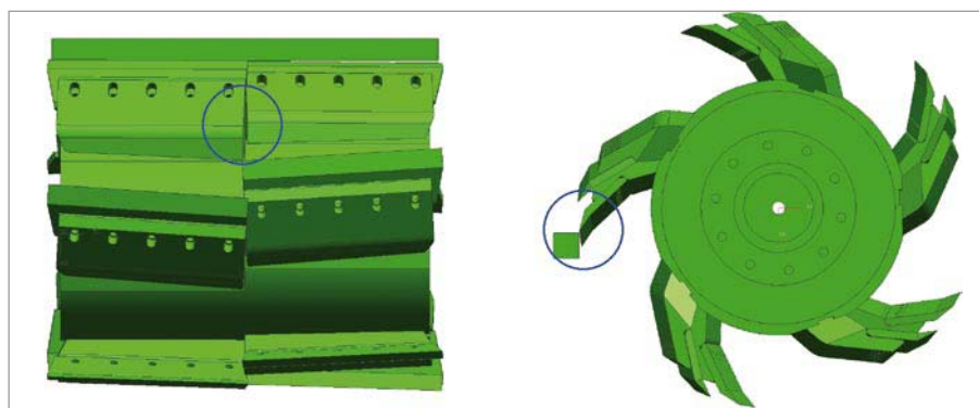
Figura 2 - Rotore CRA-ING di seconda generazione.
