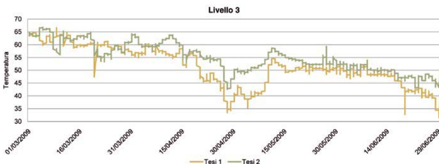
Grafico 5 - Temperatura interna dei due cumuli al livello 3.
