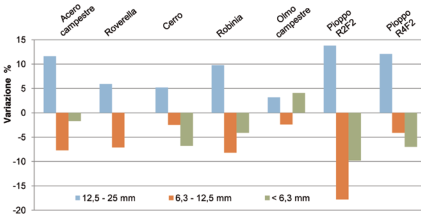
Grafico 1 - Variazione percentuale della distribuzione granulometrica del cippato prodotto dal rotore CRA-ING, rispetto al rotore Claas Jaguar, per le classi più rappresentative.
