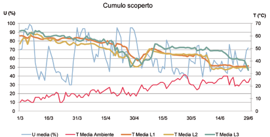
Grafico 2 - Diagramma rappresentativo delle medie delle temperature interne del cumulo scoperto.
