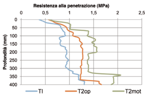
Grafico 2 - Valori medi della resistenza alla penetrazione nel cantiere falciatrici-caricatrice Spapperi.
