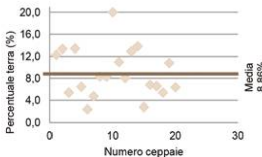
Grafico 2 - Sistema GDC - percentuale di terra rimasta sulle ceppaie di vite estratte dalla macchina.
