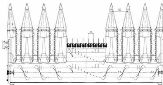
Figura 5 - Testata vista dall'alto, in evidenza le catene trasportatrici per il convogliamento dei capolini.
