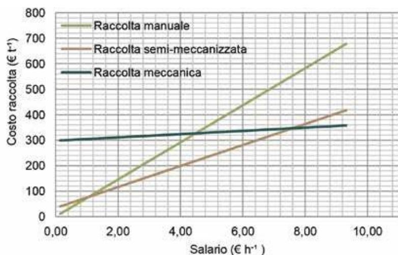
Grafico 1 - Limite di convenienza economica dei vari metodi di raccolta (manuale, semi-meccanizzato e completamente meccanizzato) nella realtà cubana.
