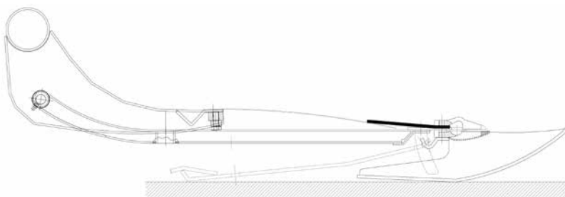
Figura 1 - Particolare falconi.
