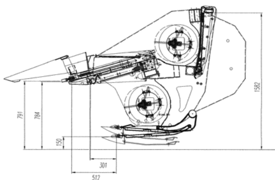
Figura 4 - Particolare della testata in sezione.
