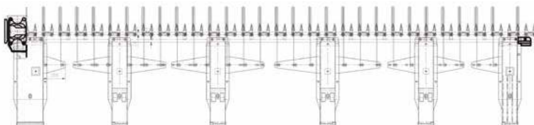
Figura 2 - Struttura mobile supportata da 6 bracci.
